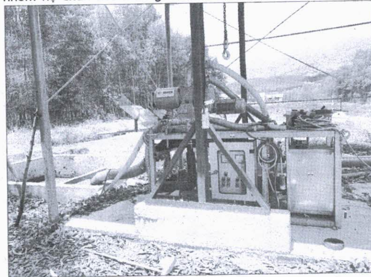
Máy tách phân được đặt trước hầm biogas của trang trại nuôi 2.000 heo nái sinh sản của ông Nguyễn Hải Đào
